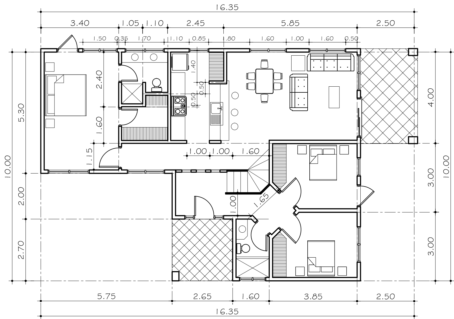
PLANTA CONSTRUCTIVA ARQUITECTONICA
