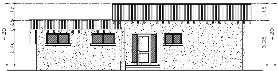
ELEVACION FRONTAL
