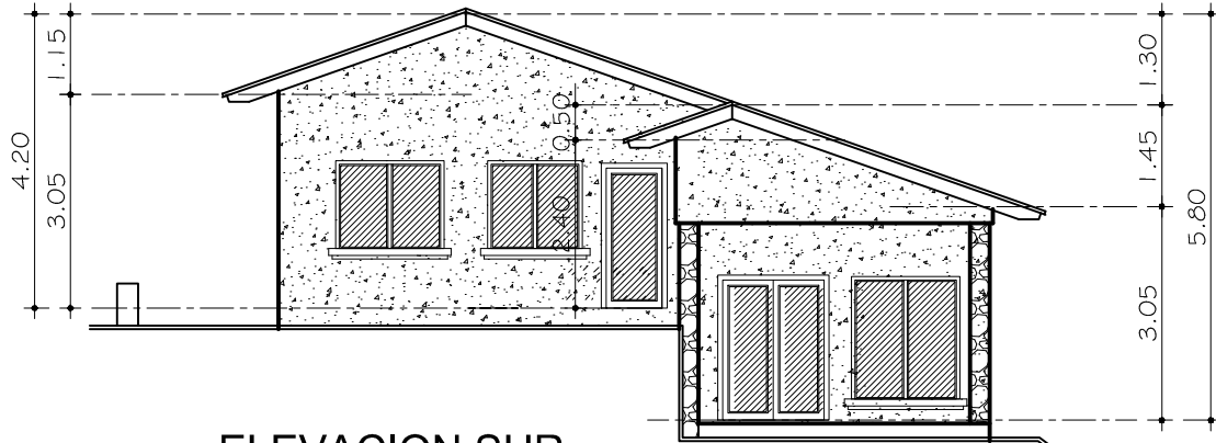
ELEVACION SUR
